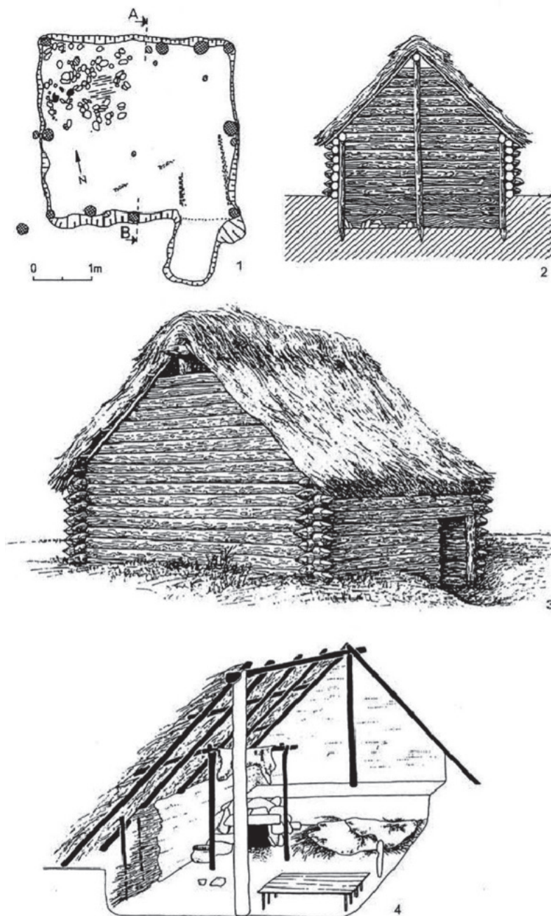
Afbeelding 10. Reconstructies van Grubenhäuser gevonden in Desau-Mosigkau (Saksen, Duitsland, nr. 1-3) en Rostoky (Tsjechië, nr. 4). Bron: Sebastian Brather, Archäologie der westlichen Slawen: Siedlung, Wirtschaft und Gesellschaft im früh- und hochmittelalterlichen Ostmitteleuropa , Berlijn/New York (2008).
